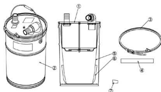
スラリーコレクター SC-25
