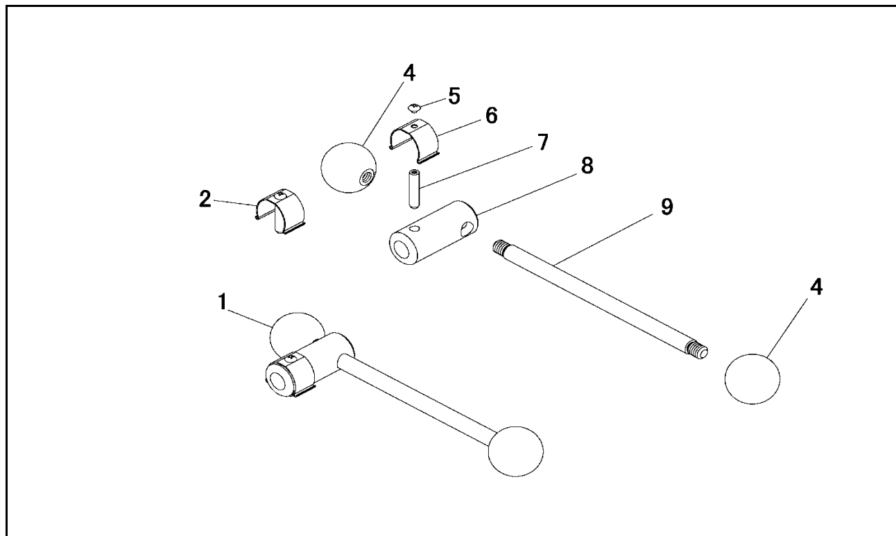
TS-605/TS-605PRO φ45ワンタッチハンドル 部品構成図
