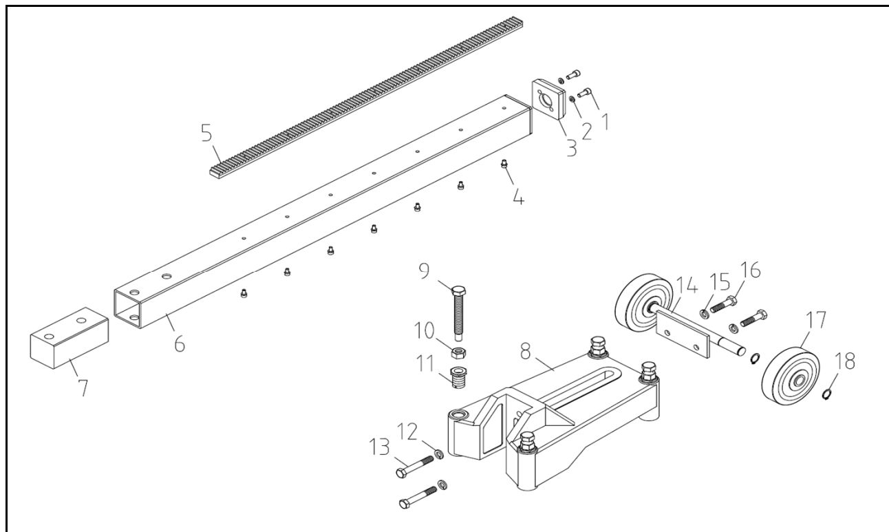
TS-605/TS-605PRO 支柱・ベース部品構成図
