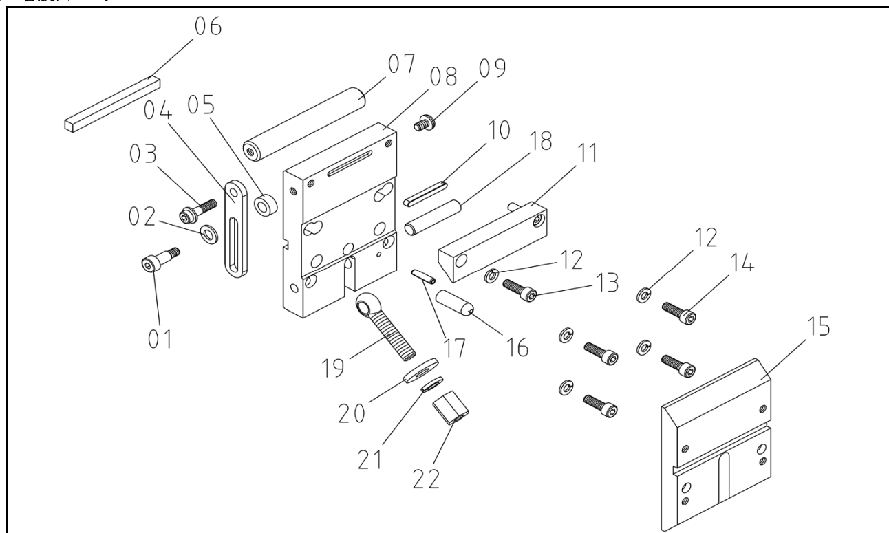
TS-605/TS-605PRO 着脱スペーサー 部品構成図
