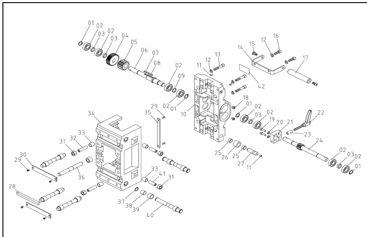
TS-605/TS-605PRO スライドブロック 部品構成図
