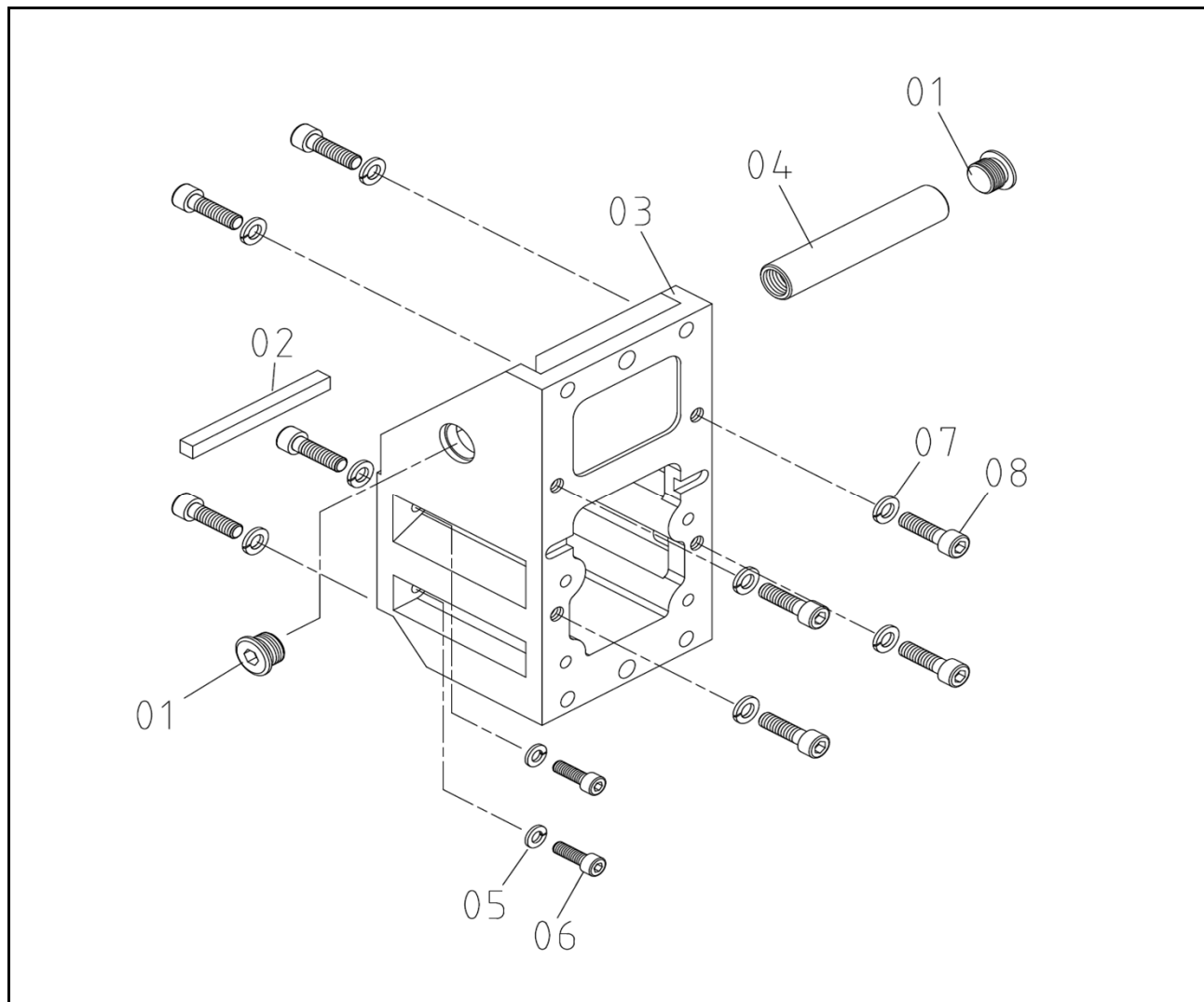
TS-605/TS-605PRO 130mmスパーサー 部品構成図
