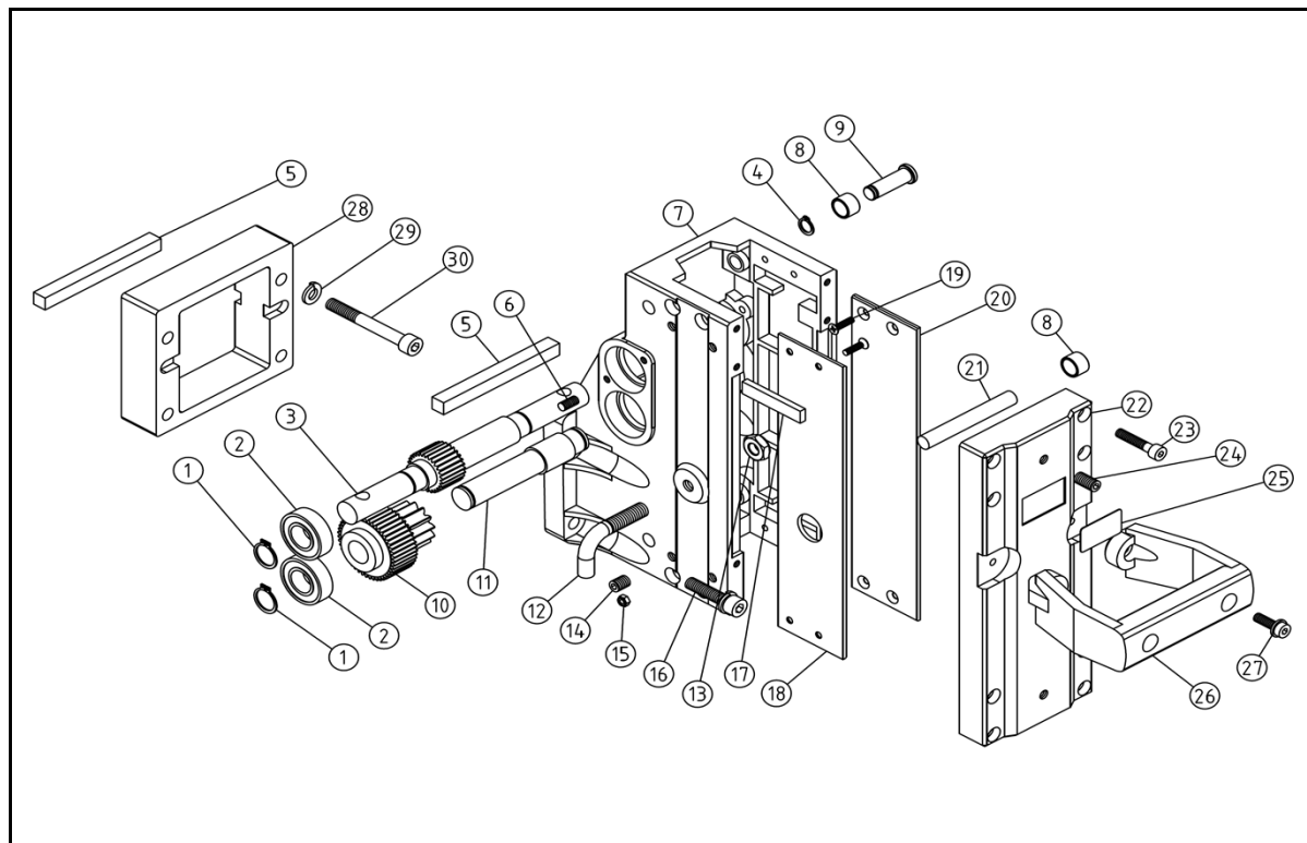
TS-405Ⅲ/TS-405PROⅢ スライドブロック 部品構成図
