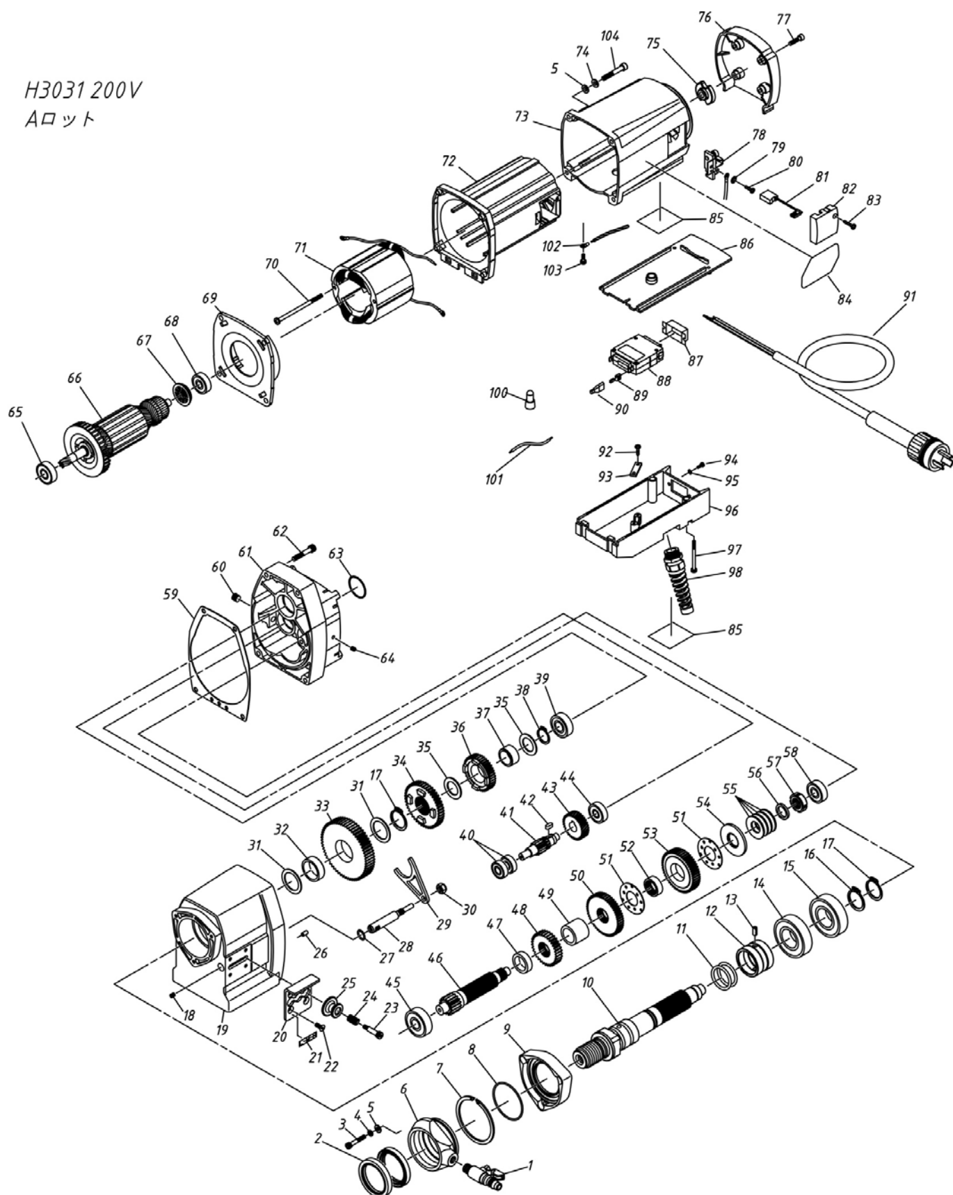
H3031 200V Aロット 部品構成図
