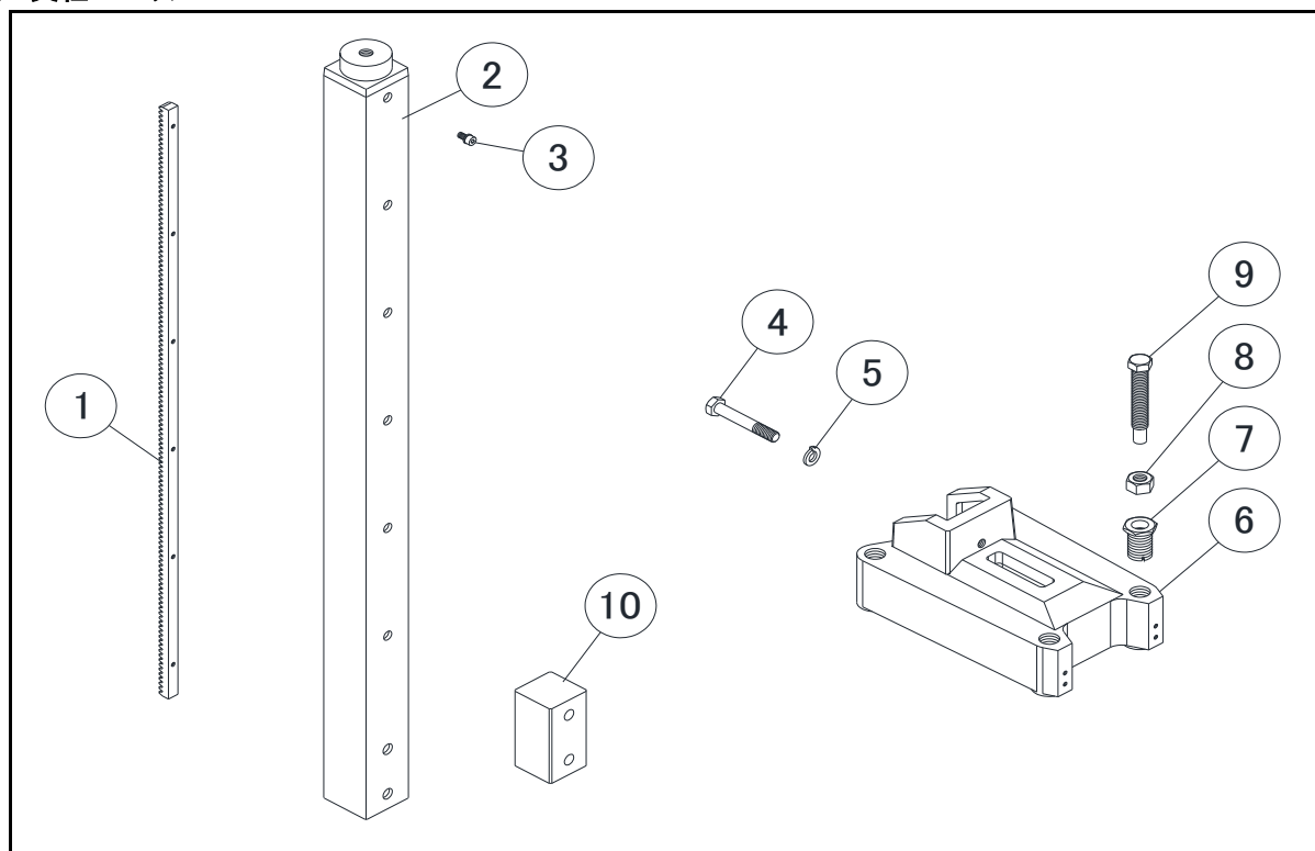
TS-405Ⅲ/TS-405PROⅢ 支柱・ベース部品構成図
