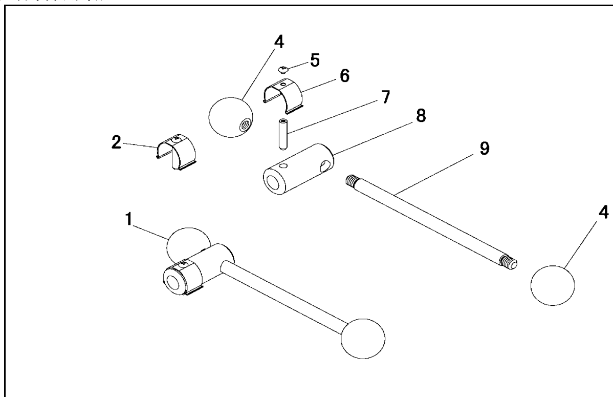
TS-405Ⅲ/TS-405PROⅢ φ45ワンタッチハンドル 部品構成図
