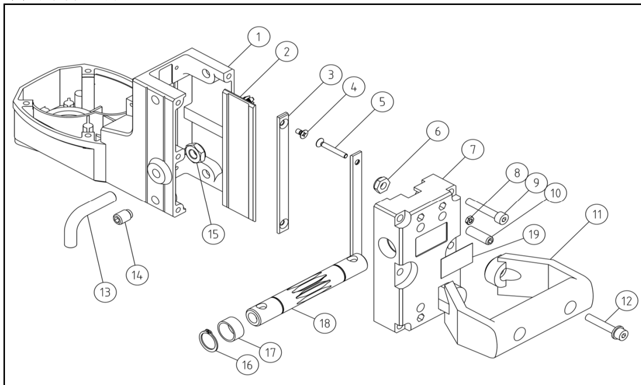
TSK-095 スライドブロック 部品構成図
