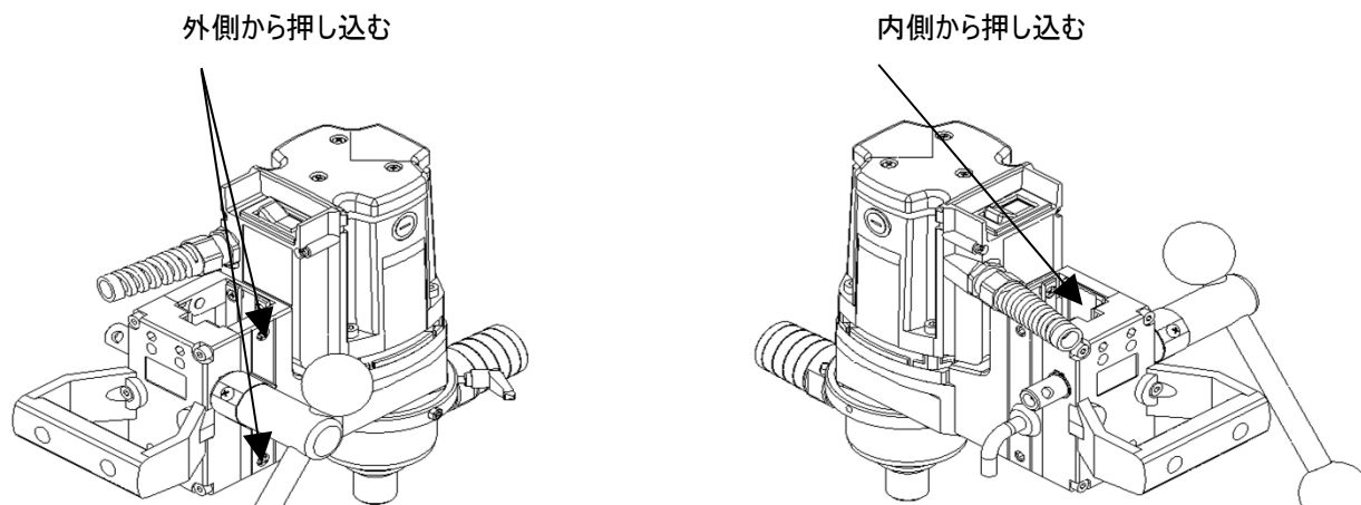
図9.3 スライドプレートの交換
