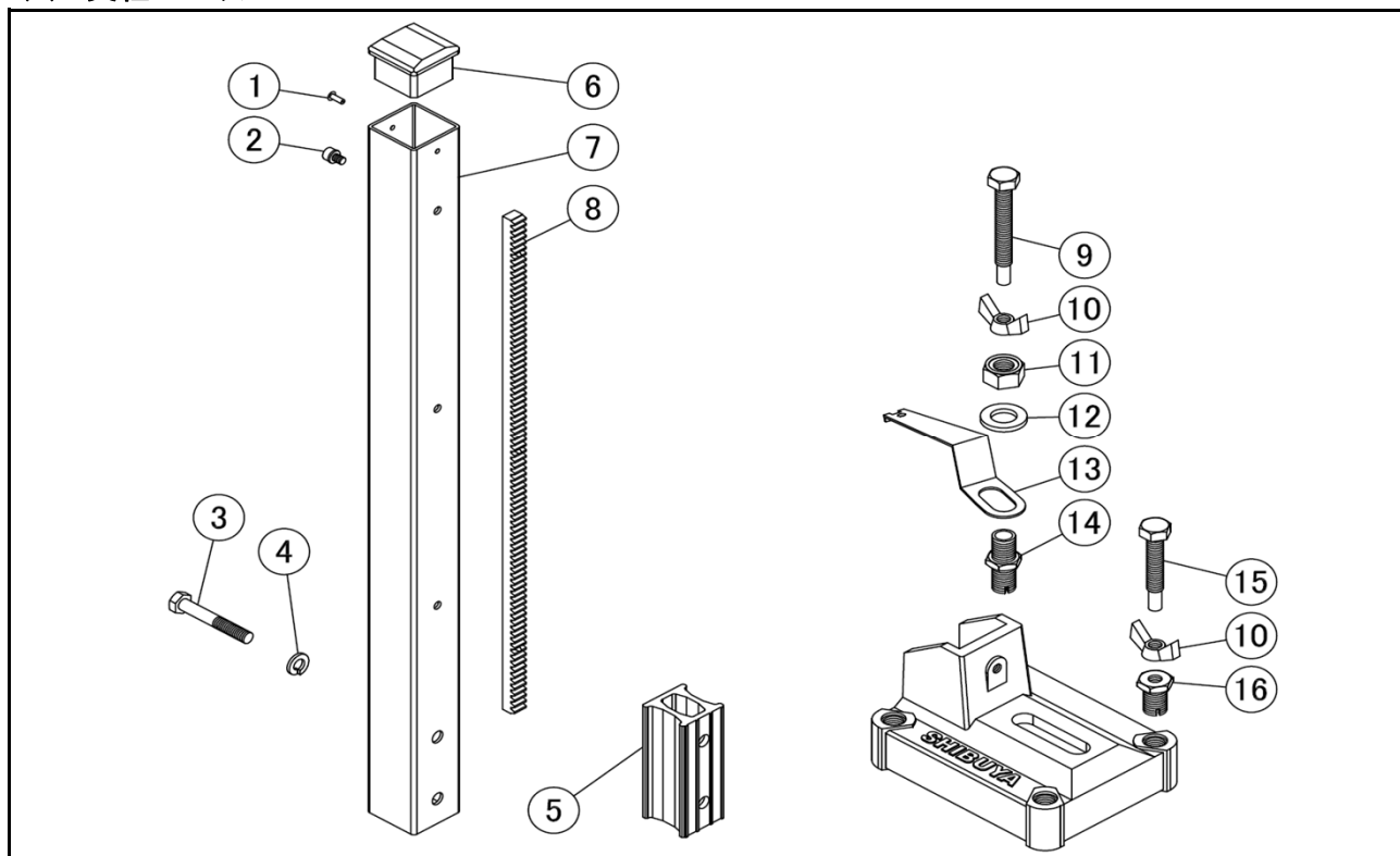
TS-095/TSC-095 支柱・ベース 部品構成図
