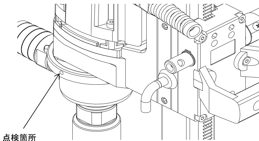
図9.4 水漏れ・エアリークの点検箇所
