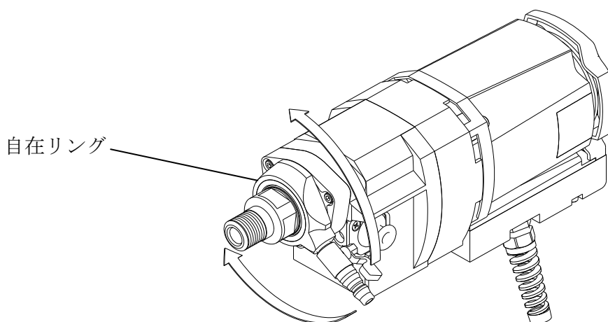
図2-2 給水部
