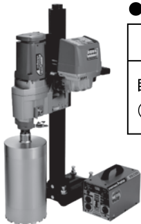
TS-405PRO+ ダイモトランス + AFS-P 仕様
