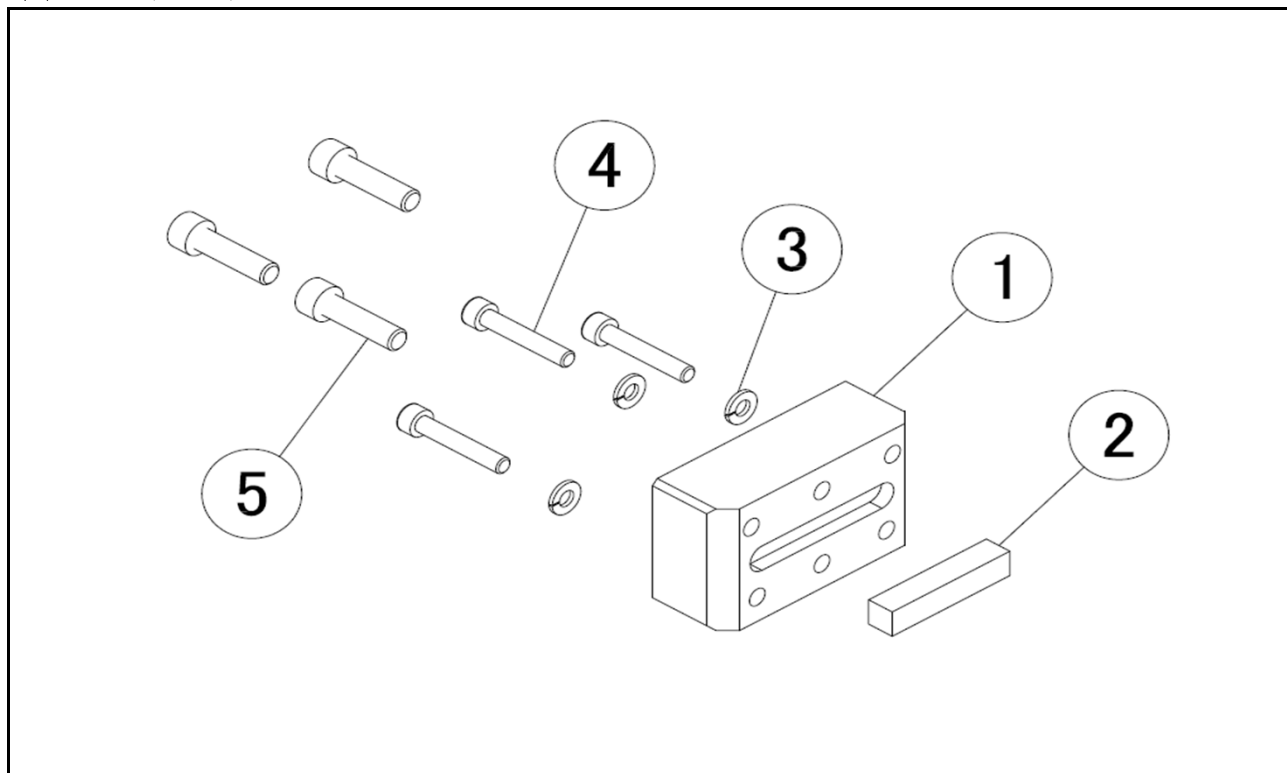
TSH-165 30mmスペーサー 部品構成図
