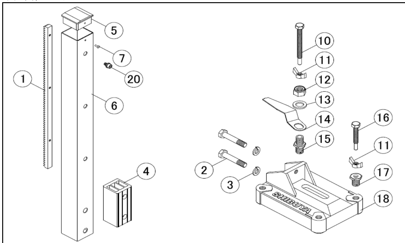
TSK-165 支柱・ベース部品構成図
