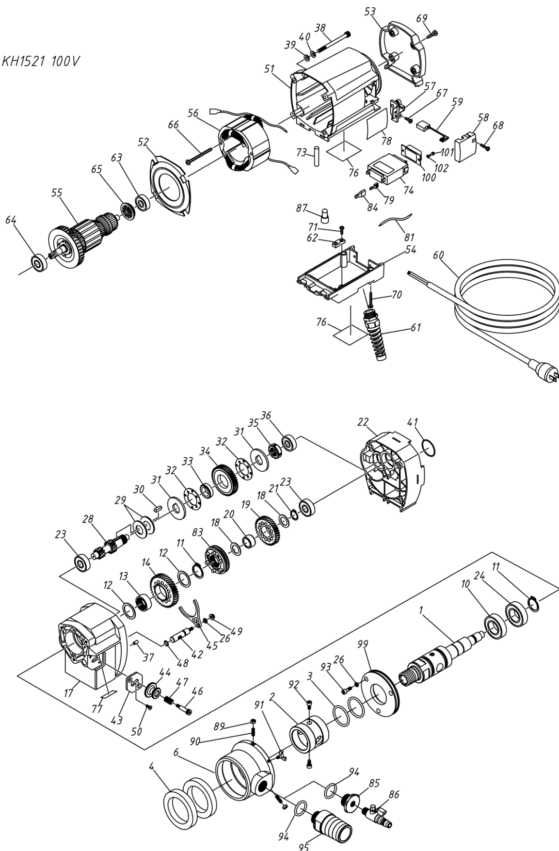
KH1521 100V 部品構成図
