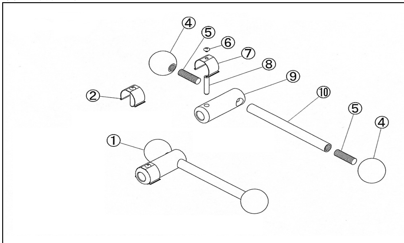
TSK-165 φ45ワンタッチハンドル(アルミ) 部品構成図
