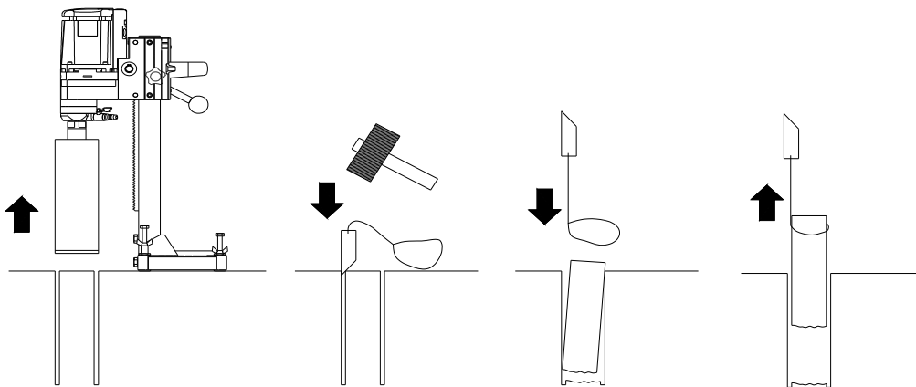
図7.11.5 コアの引き抜き
