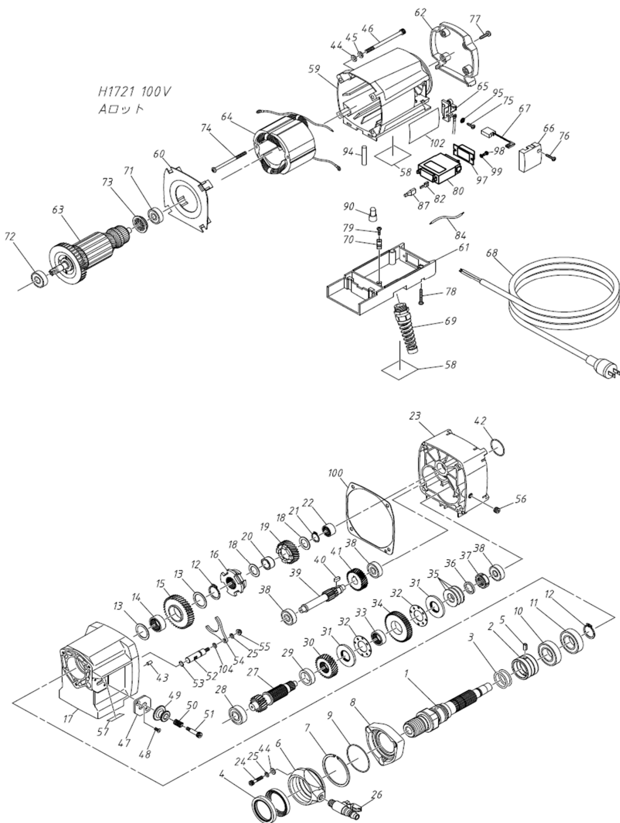
H1721 100V Aロット 部品構成図
