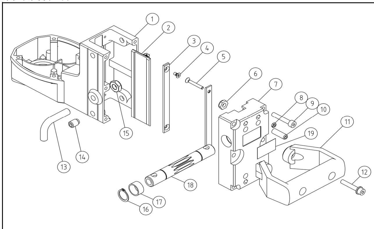
TS-095/TSC-095 スライドブロック 部品構成図
