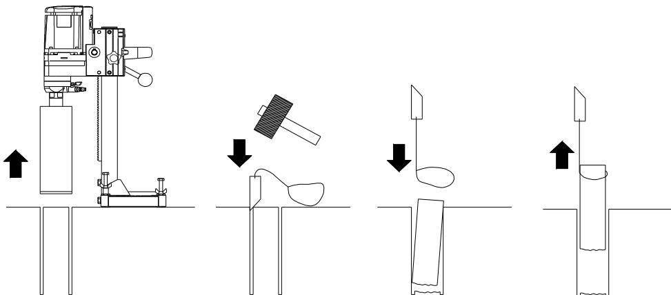
図7.7.5 コアの引き抜き
