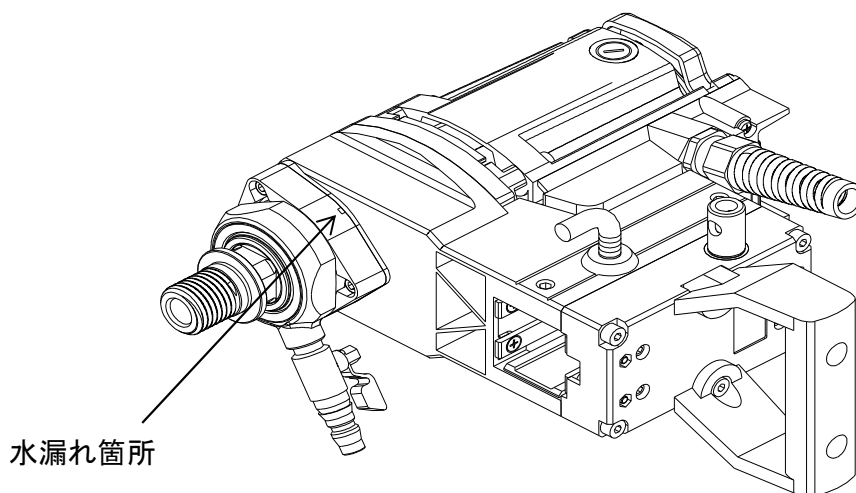
図9.4 水漏れの点検箇所
