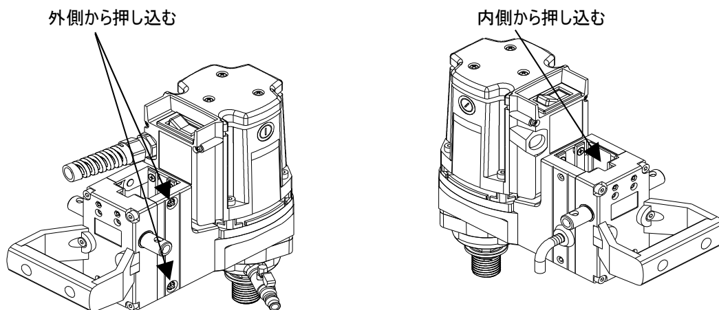
図9.3 スライドプレートの交換
